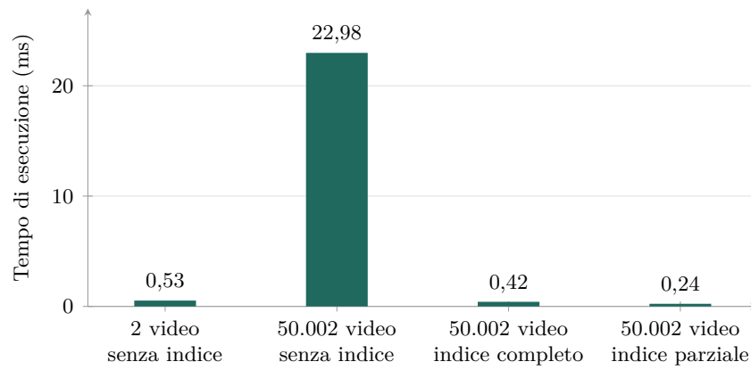
Figura 2: Costo dell'interrogazione del feed pubblico nelle quattro configurazioni misurate. Senza indice il tempo cresce con la dimensione del catalogo; l'indice parziale lo riporta sotto il quarto di millisecondo.
